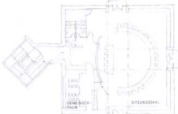
Grundriss 2. Obergeschoss
